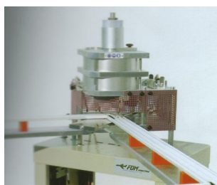
Sertisseuse verticale
