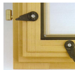
Clips tournante
